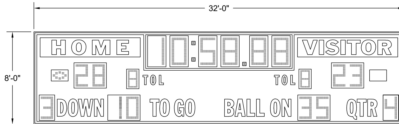
FB-8132TKH-2
