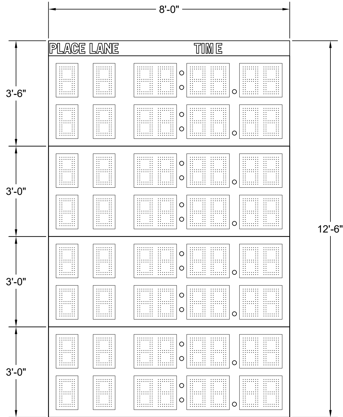
TK-1508-V-2
