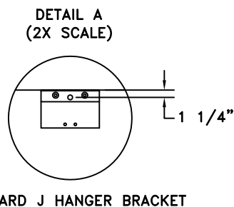
DIMENSIONS FB-8114-2
